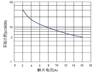
电寿命曲线图
