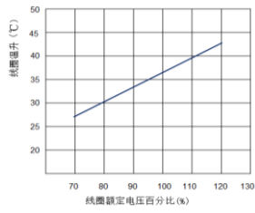
线圈温升曲线图
